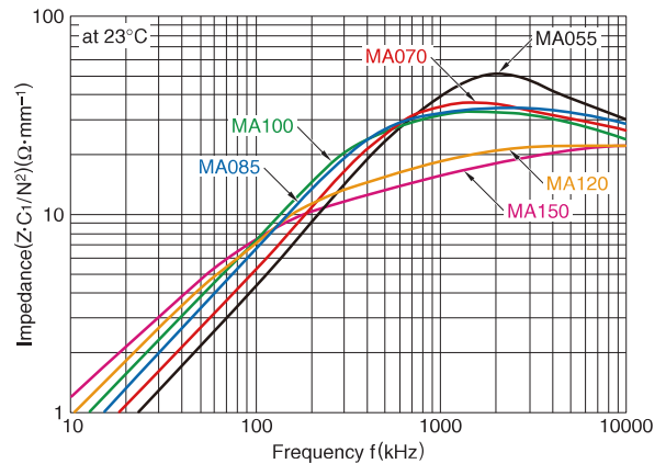
インピーダンス(Z·C1/N 2 )-周波数特性 Impedance(Z·C1/N 2 ) vs. Frequency(Typical)
